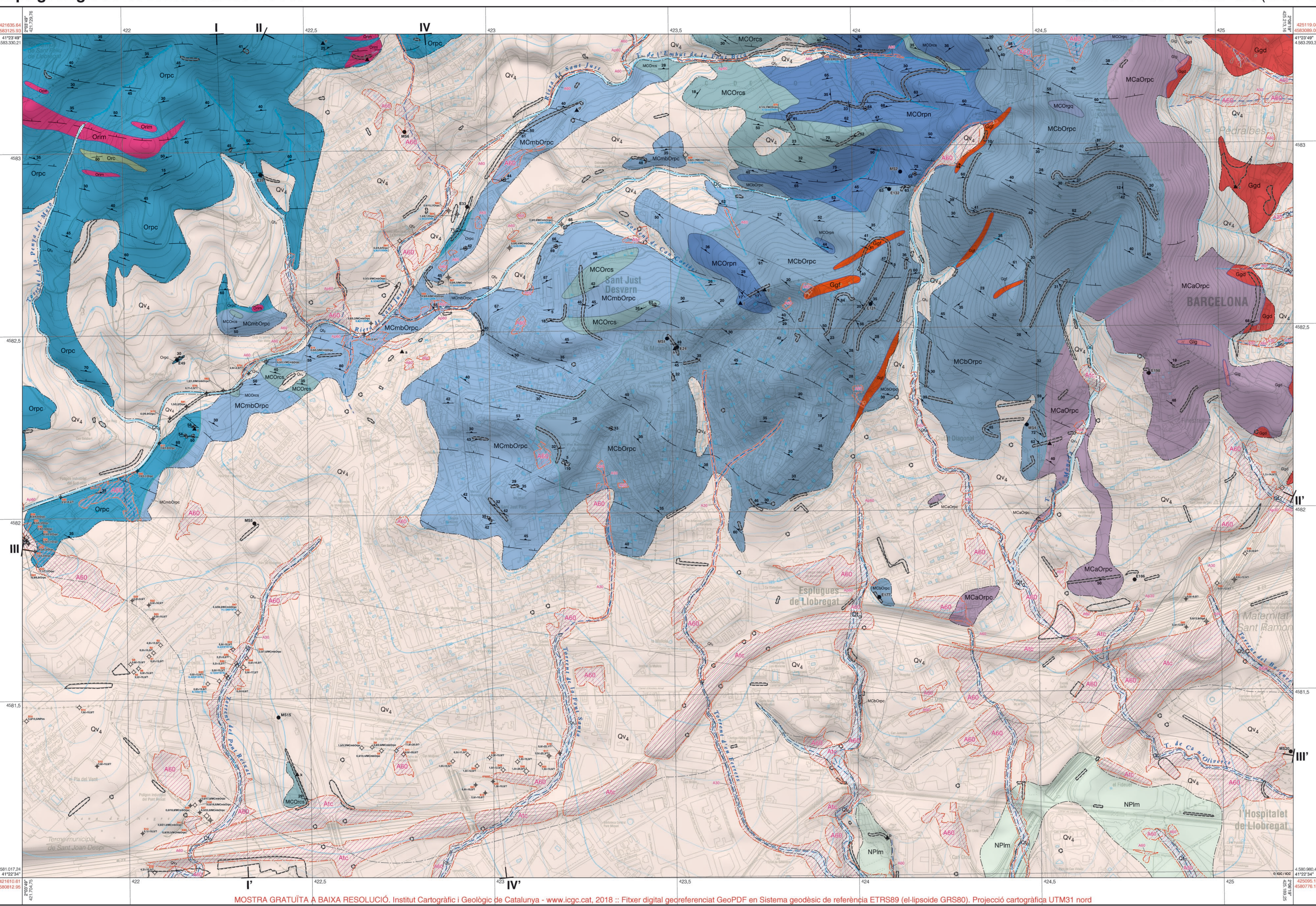
MOstra GRATUÏTA A BÀIXA RESOLUCIÓ. Institut Cartogràfic i Geològic de Catalunya - www.icgc.cat - Fitxer digital geològic GeoPDF en el Sistema de Gestió de Referència ITRRS89 del tipus GRS03. Projecció cartogràfica UTM31 nord
