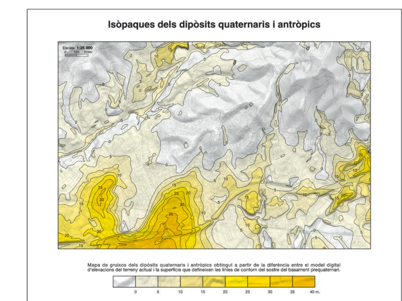
MOstra GRATUÏTA A BÀIXA RESOLUCIÓ. Institut Cartogràfic i Geològic de Catalunya - www.icgc.cat - Fitxer digital geològic GeoPDF en el Sistema de Gestió de Referència ITRRS89 del tipus GRS03. Projecció cartogràfica UTM31 nord
